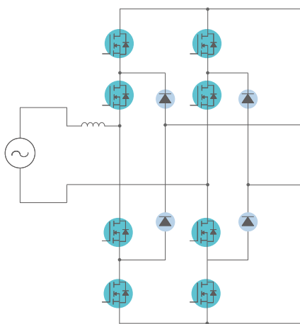
全桥三电平
